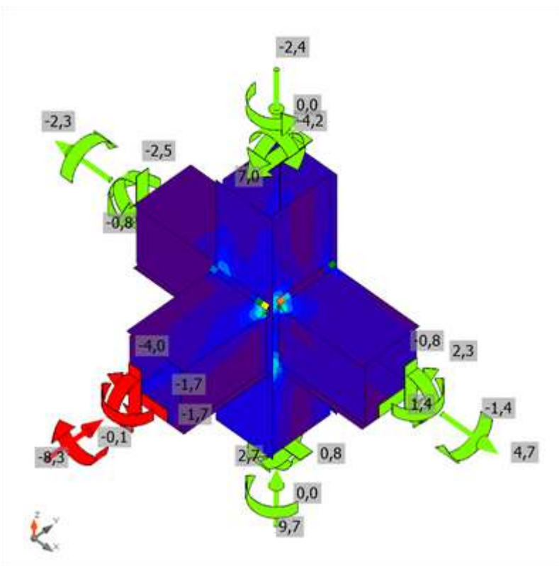
Sforzo equivalente, SLU 123(1)
